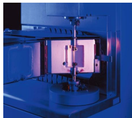
Testen van kunststoffen
